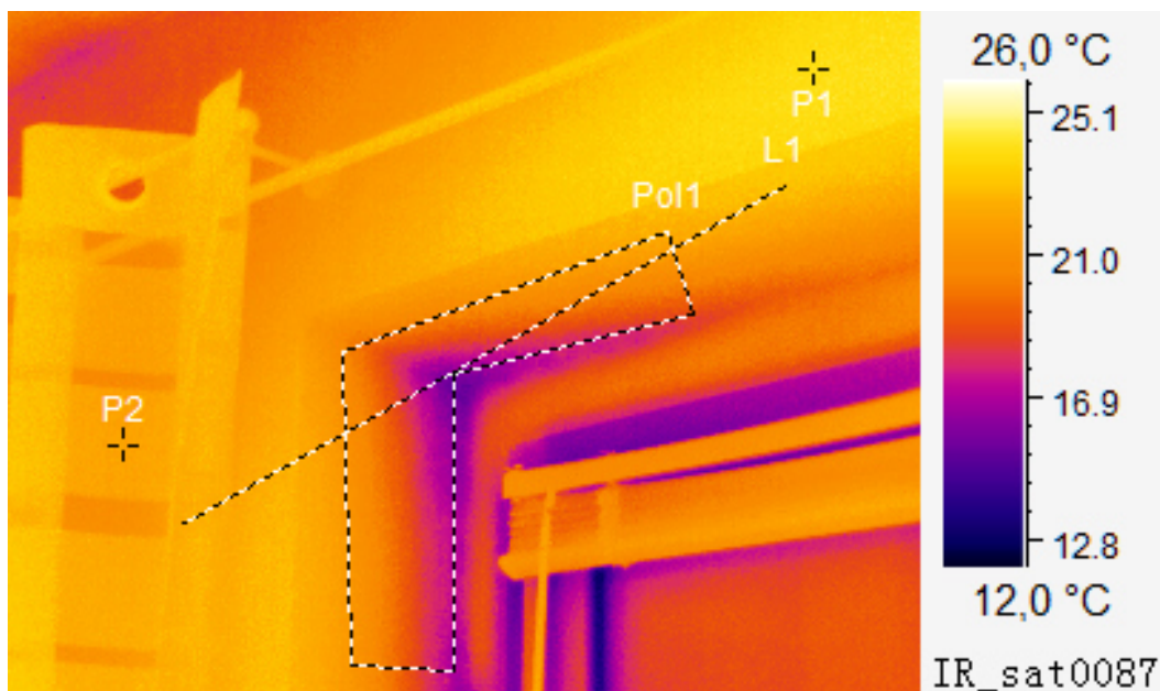
Abb.5: Wohnen, linkes Fensterelement – Anschluss linke Laibung/Sturz
